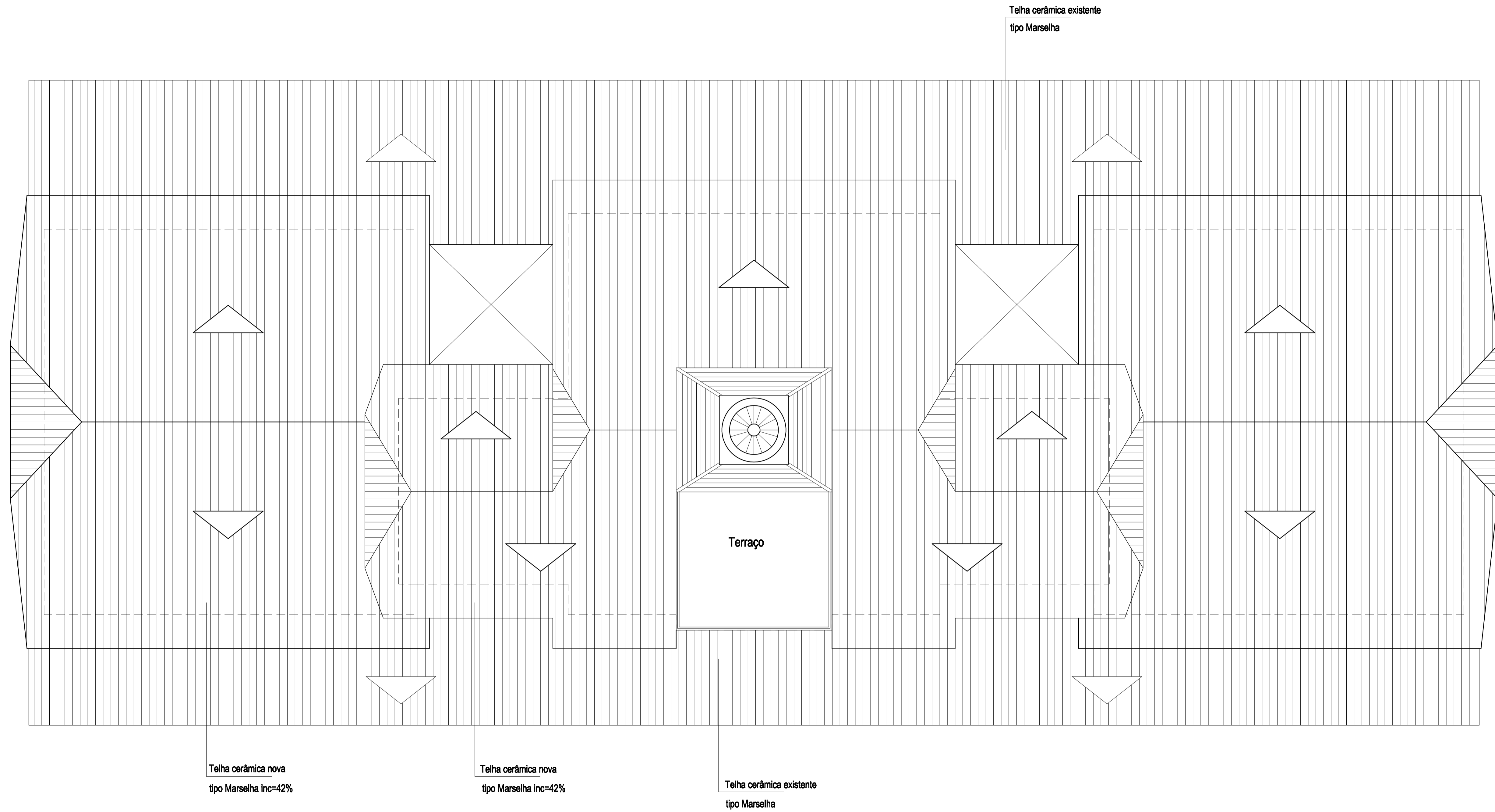
01 PLANTA DE COBERTA ESC. 1/75
