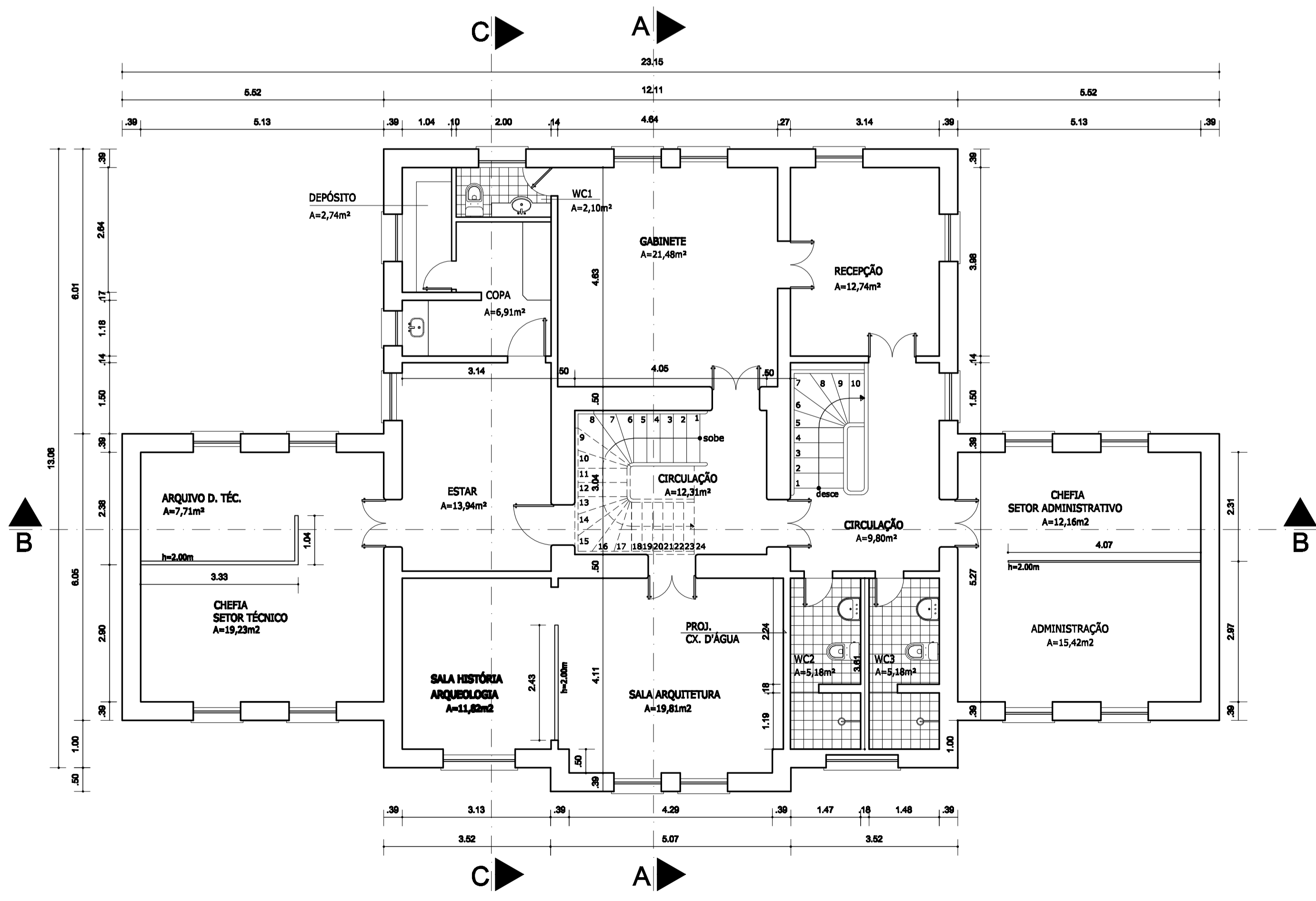
02 PLANTA BAIXA PAV. SUPERIOR ESC. 1/75
