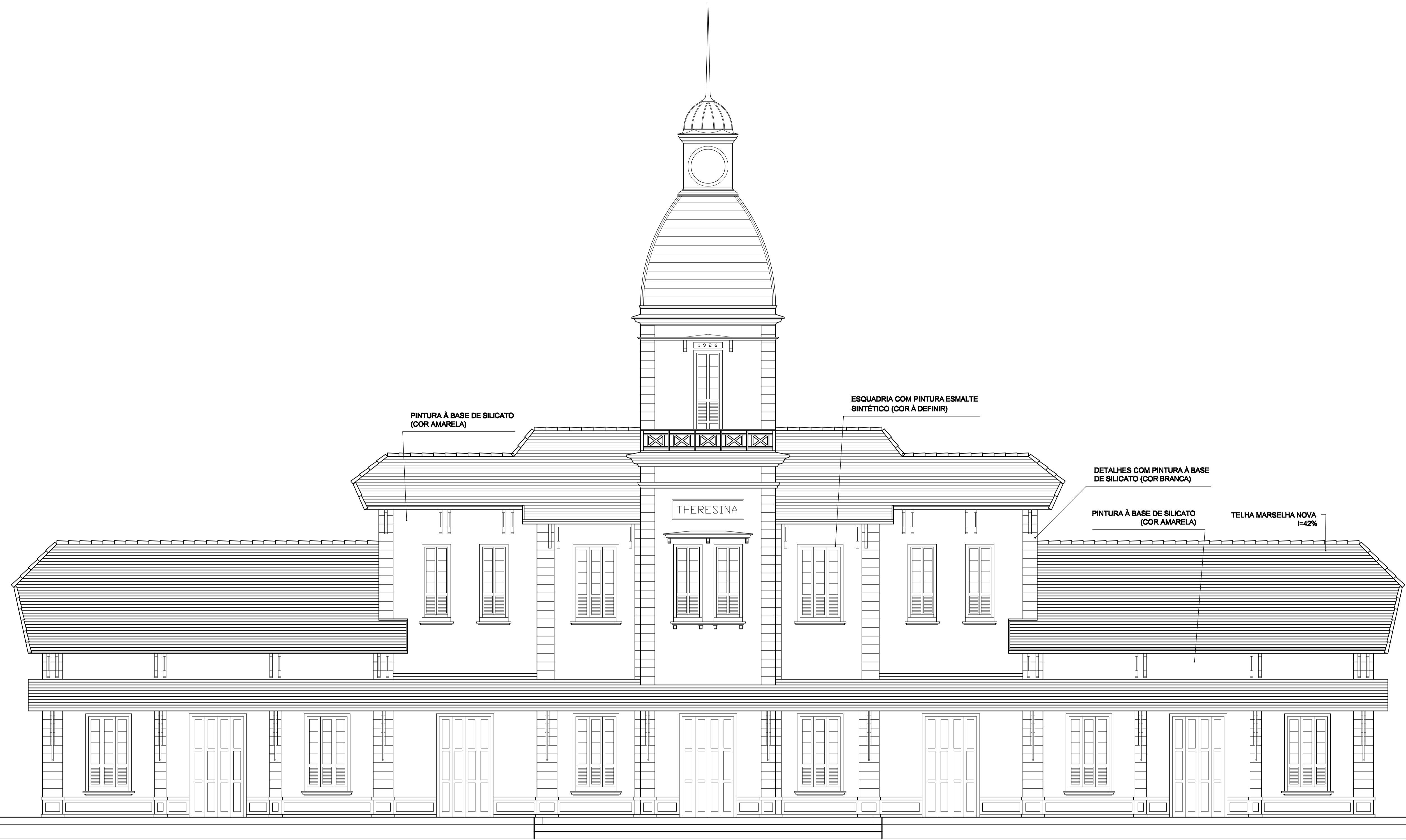
01 ELEVÇÃO PRINCIPAL ESC. 1/75
